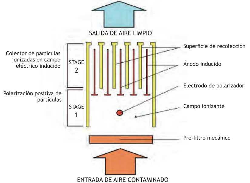
Principio operativo del filtro electrostático CrystallFEMEC SABIANA
